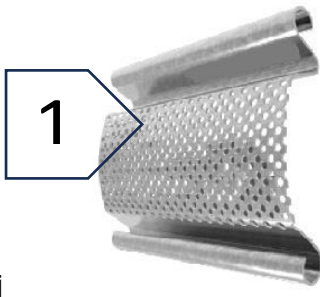
G 120 MİKRO DELİKLİ
